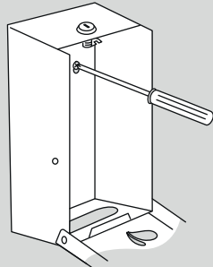
2. Faça as marcações, fure a parede, insira as buchas e fixe com os parafusos;
